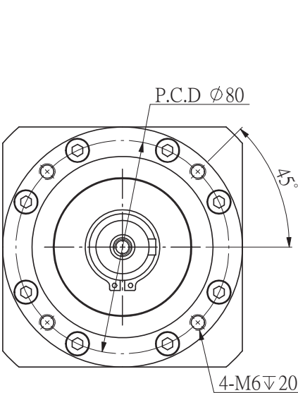
輸出端output
