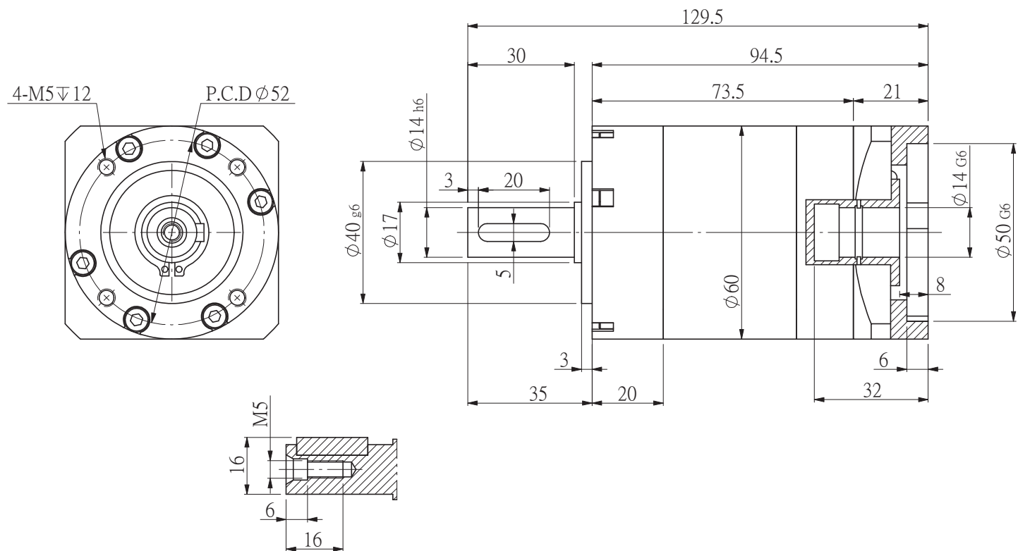
輸出端output
