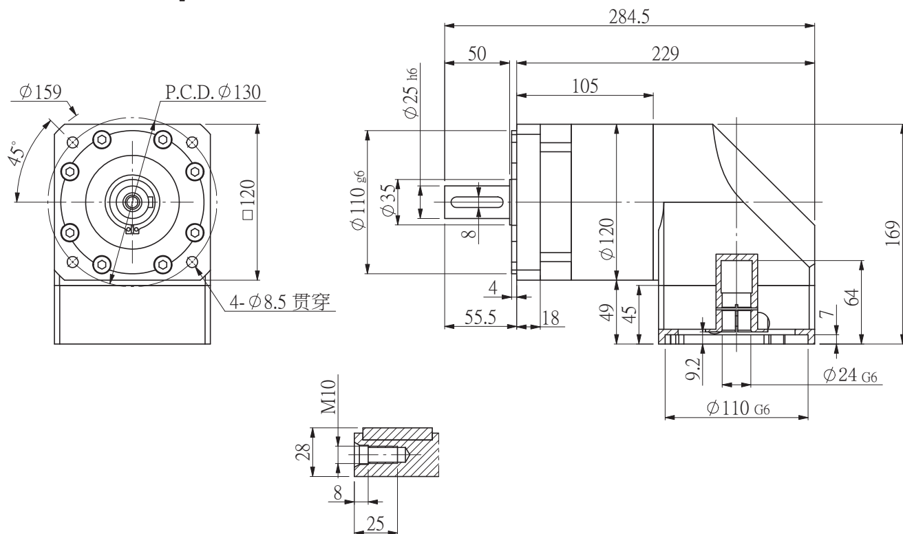
輸出端output
