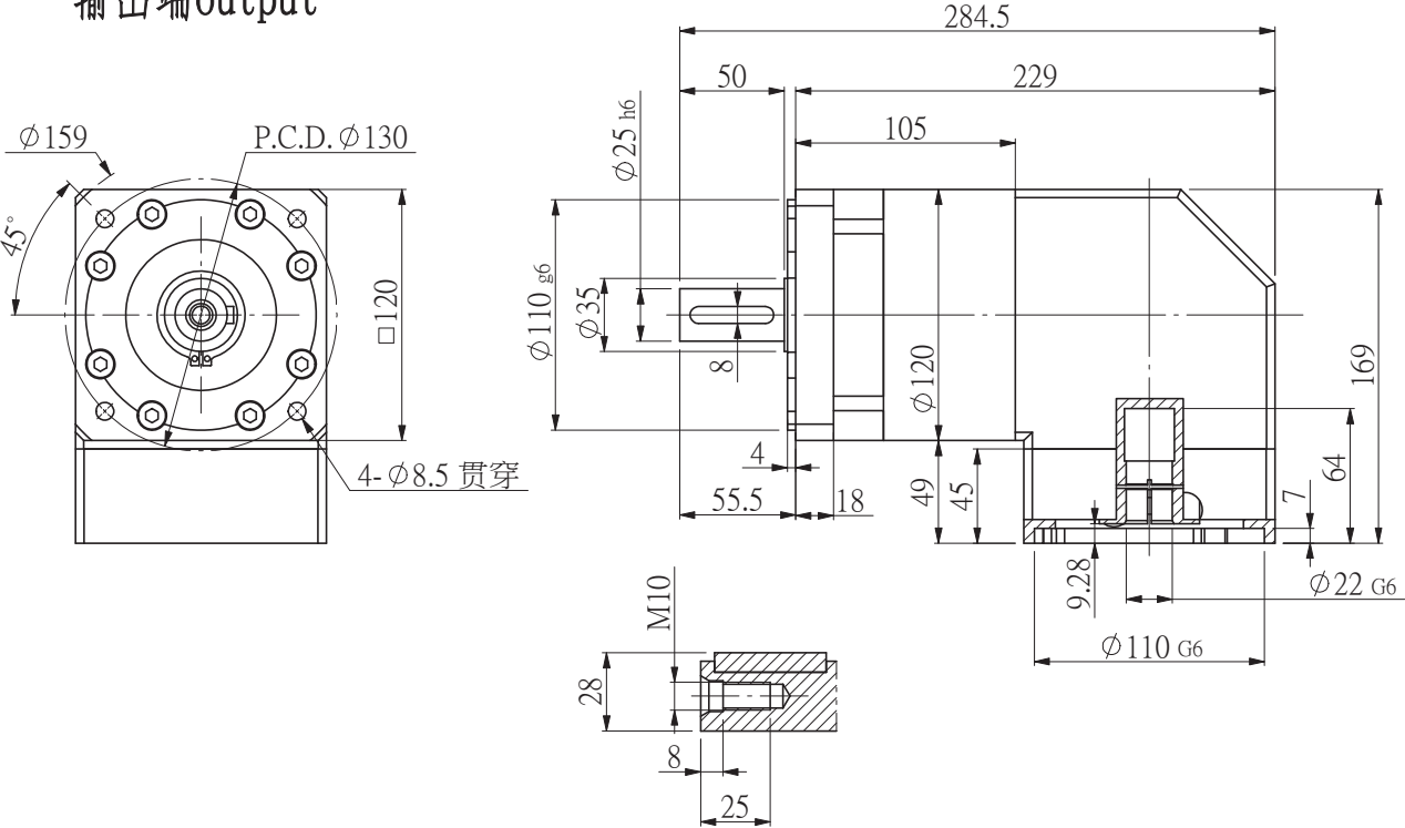
输出端output
