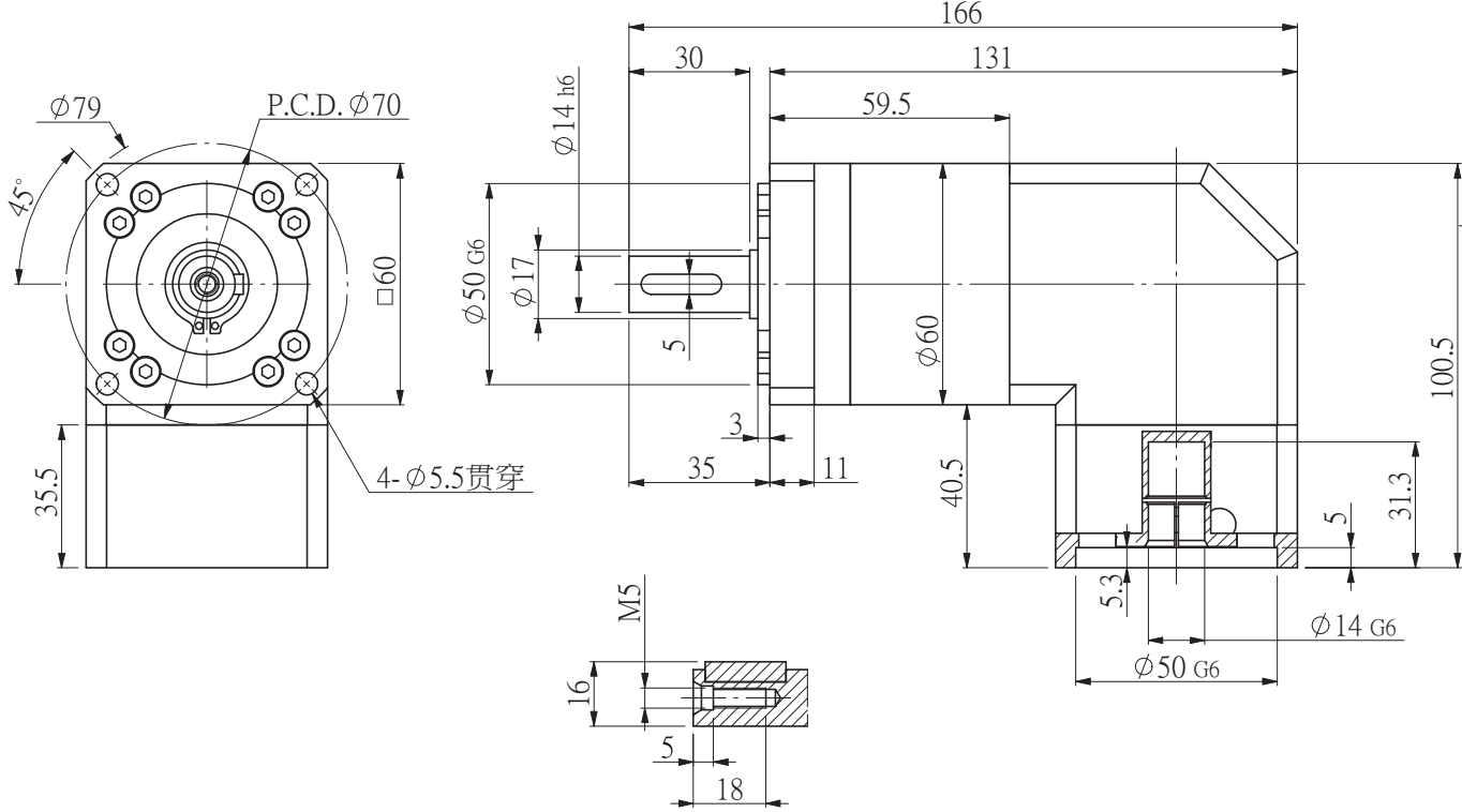
输出端output
