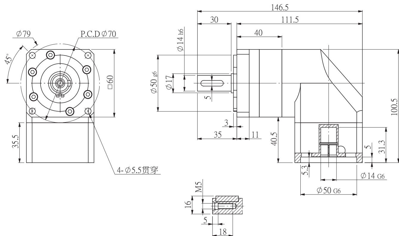
输出端output
