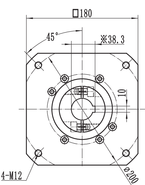
输入端input
