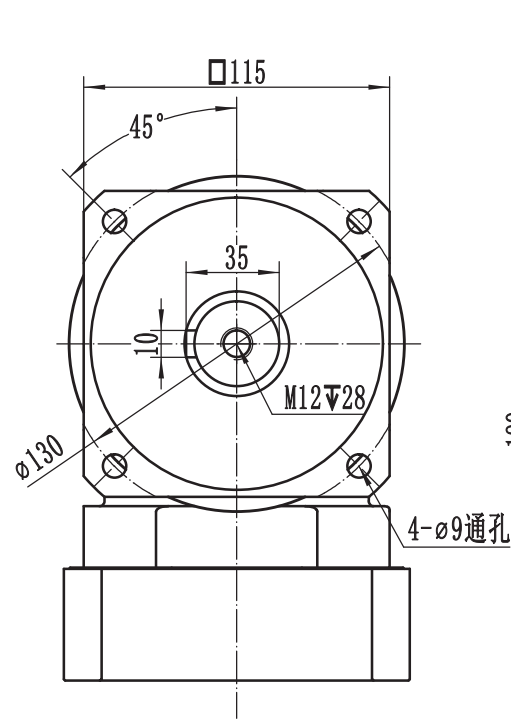
输出端output
