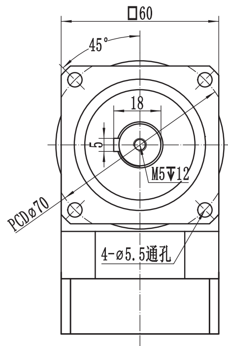
輸出端output
