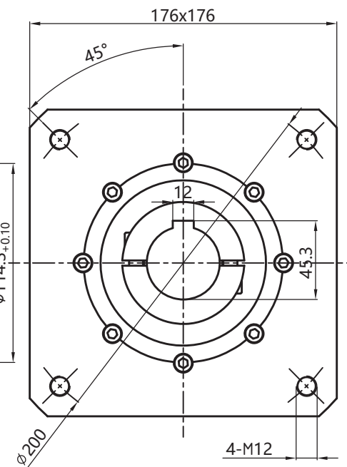
输入端input
