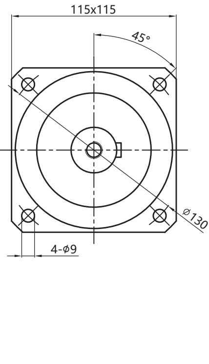
輸出端output
