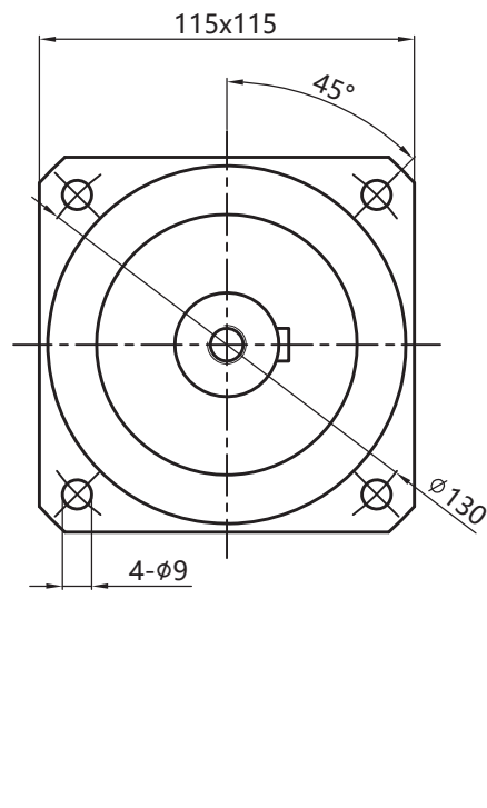
输出端output
