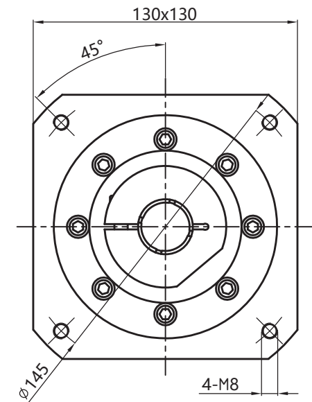
输入端input
