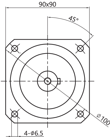
輸出端output
