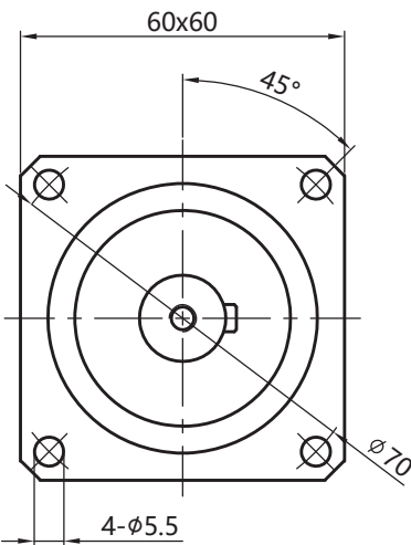
輸出端output
