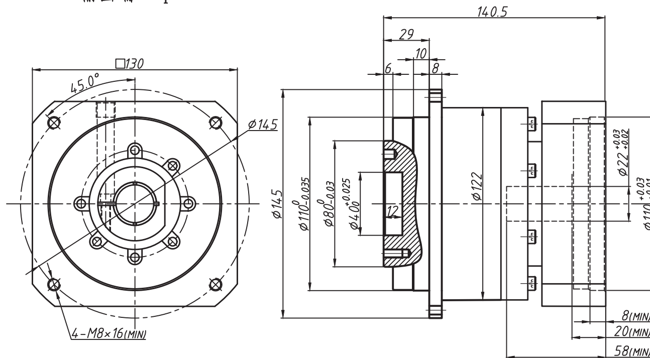
輸出端output
