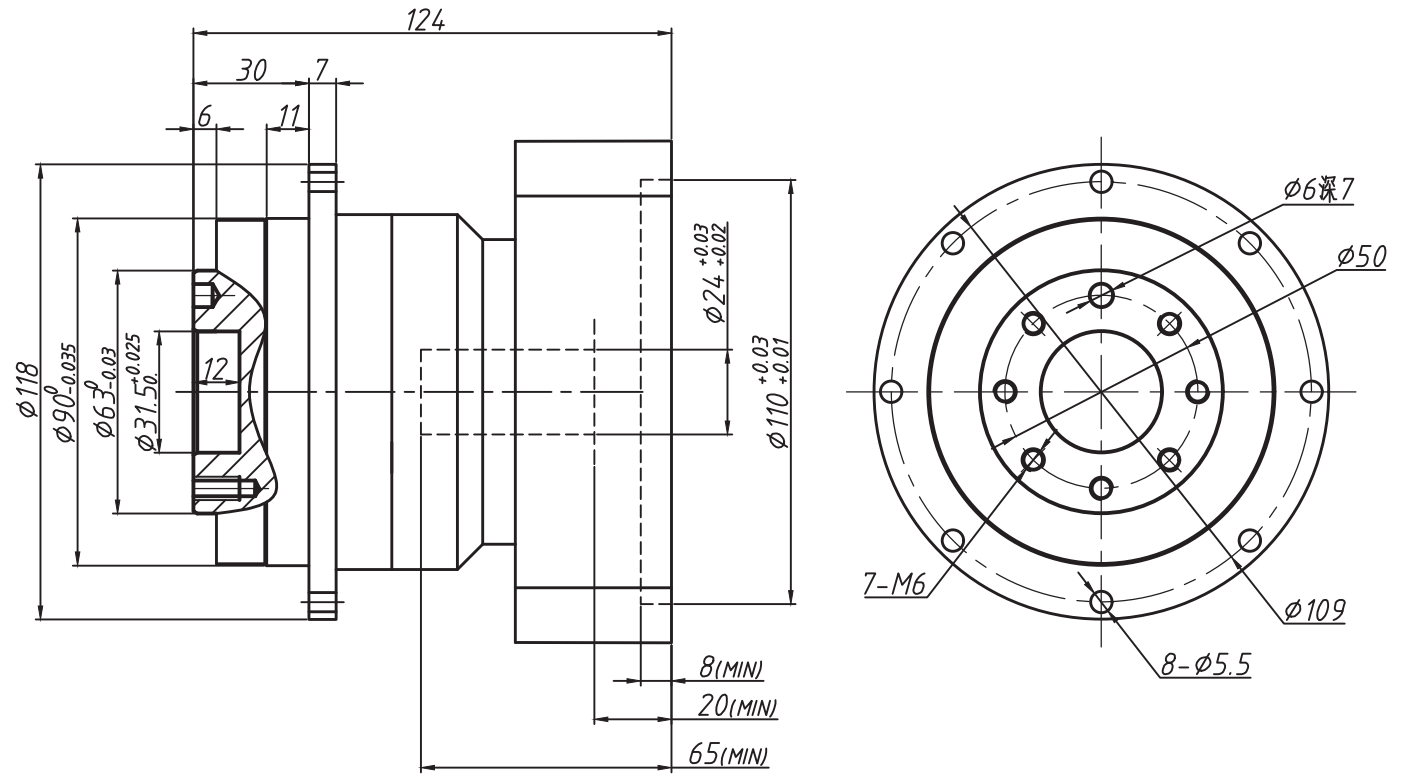
输出端output
