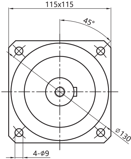
輸出端output
