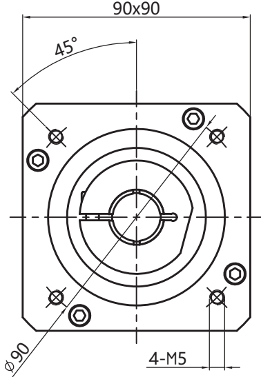
輸出端output
