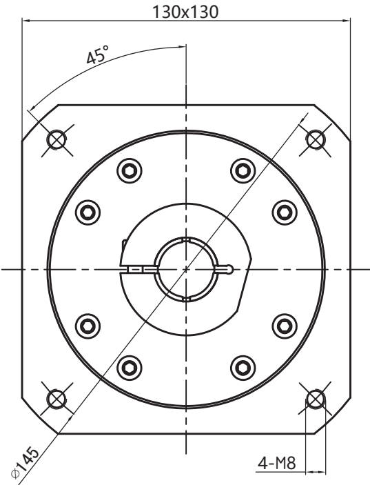
输入端input
