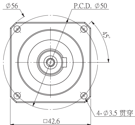
输出端output
