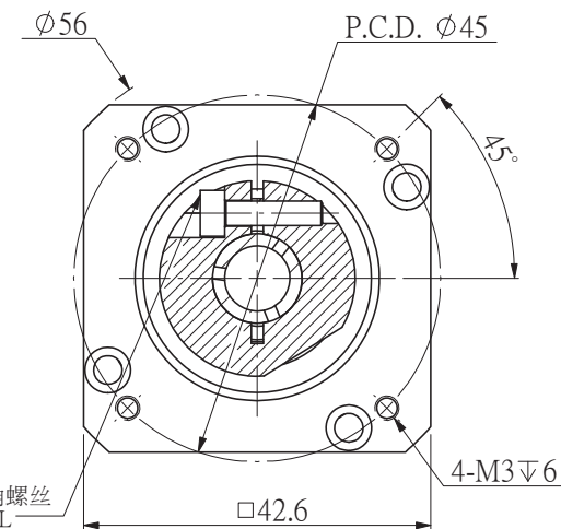
输入端input
