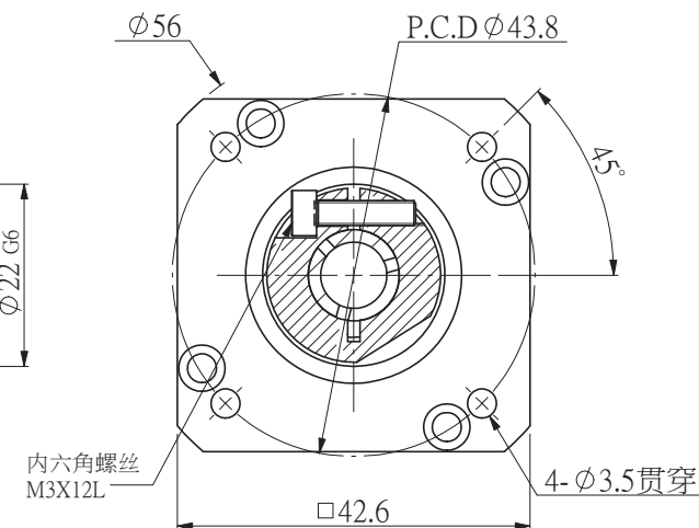
输入端input
